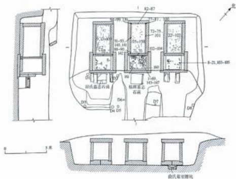
图 4-98 M11 平面、剖面图
